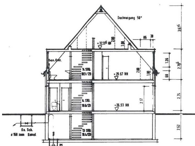
Querschnitt
